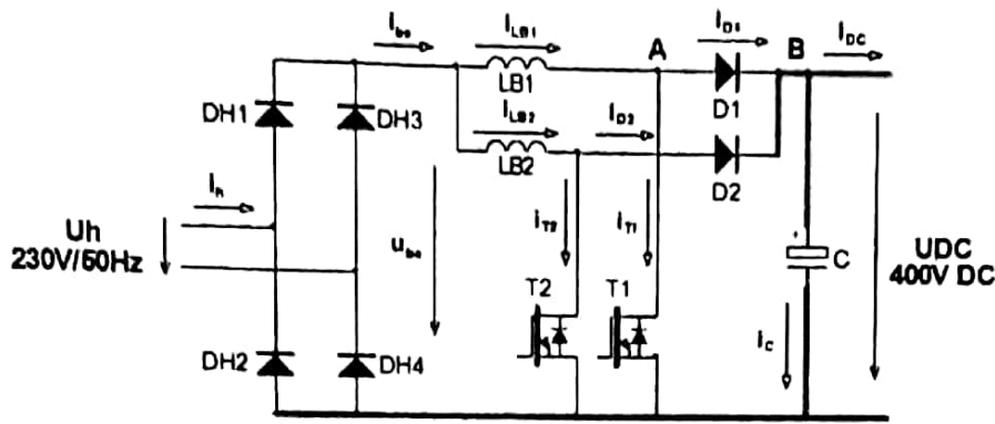
4. ábra: „Interleaved” topológiájú PFC áramkör főáramköri kialakítása
