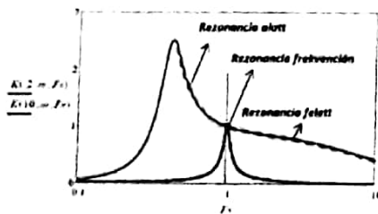
9. ábra: Reszgőkörös konverter átviteli tényezőjének frekvenciafüggése
