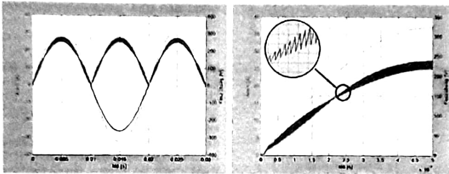
5. ábra: „Interleaved” topológiájú PFC áramkör legfőbb jelalakjai: hálózati feszültség (kék), hálózati áram (rózsaszín), booster fojtók árama a közös ágban (piros)
