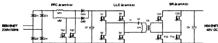
3. ábra: DHPQ típusú tápegység főáramköri kapcsolási rajza
