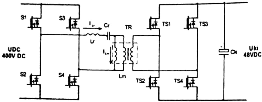
Rezgőkörös konverter
