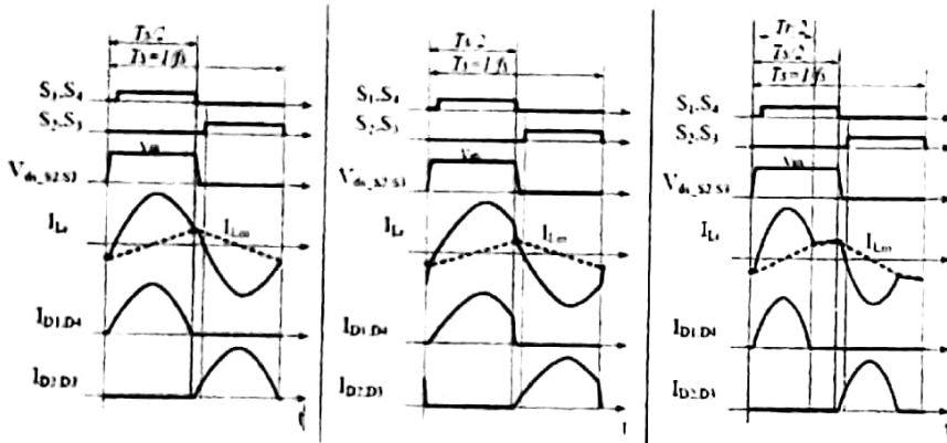
8. ábra: Reszgőkörös konverter jellemző jelalakjai
