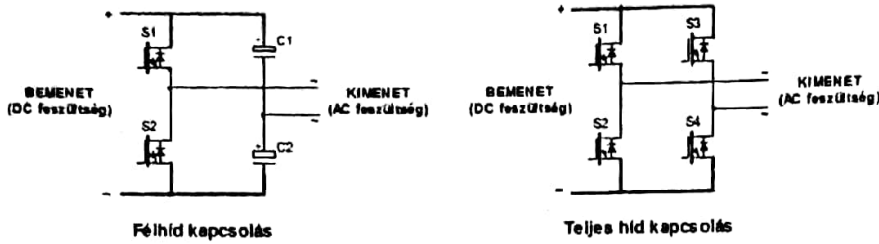
1. ábra: Rezgőkörös konverter hidkapcsolás topológiák
